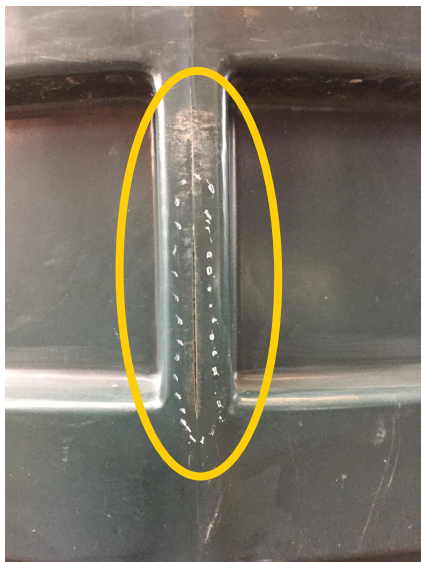
Revne opstået i forsætning ved tankens endeflade
